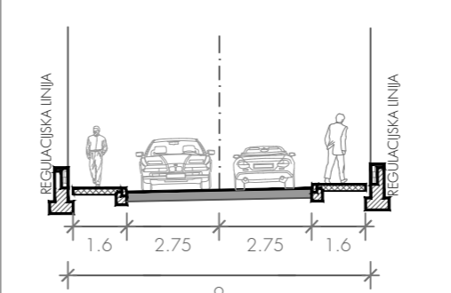
PRESJEK E-E
