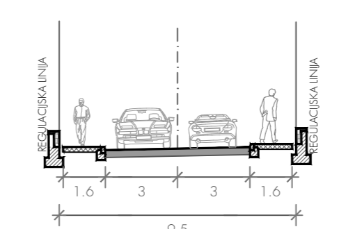
PRESJEK F-F
