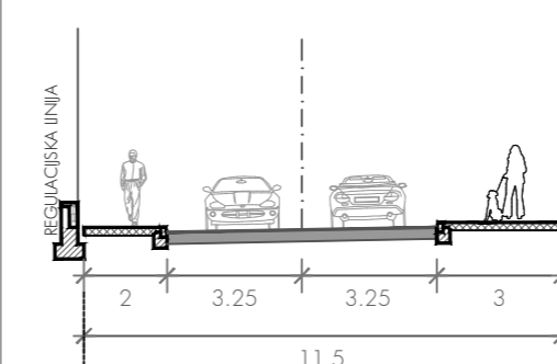
PRESJEK C-C
