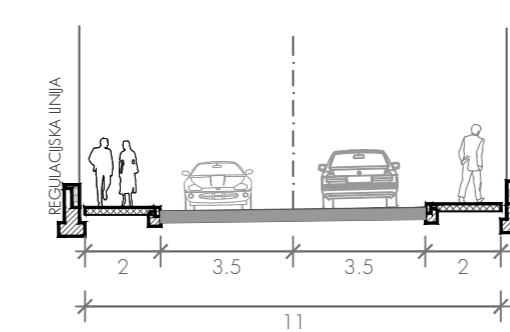
PRESJEK D-D
